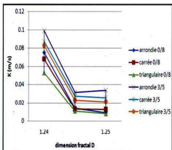
Fig .11. Courbe de perméabilité en fonction de la dimension fractale
