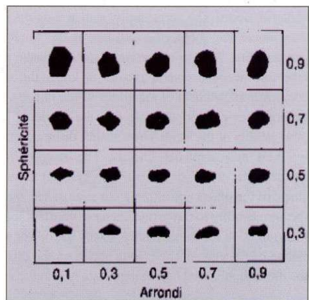
Fig.2. Indices d'arrondi et de sphéricité
