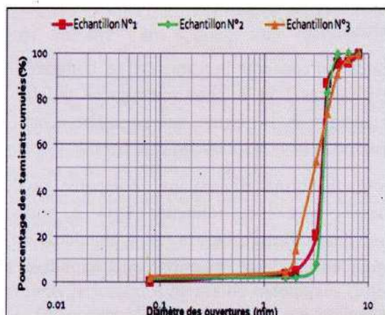
Fig. 3. Courbes granulométriques des trois types de sables étudiés
